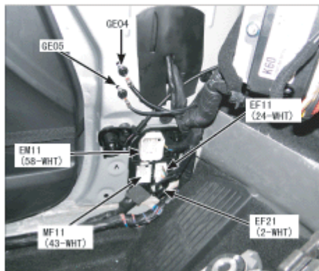
43. 左侧A-立柱底部
